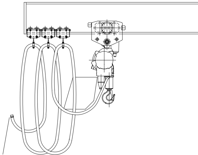
Hauptluftanschluss
