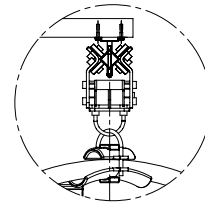
Einzelheit B
