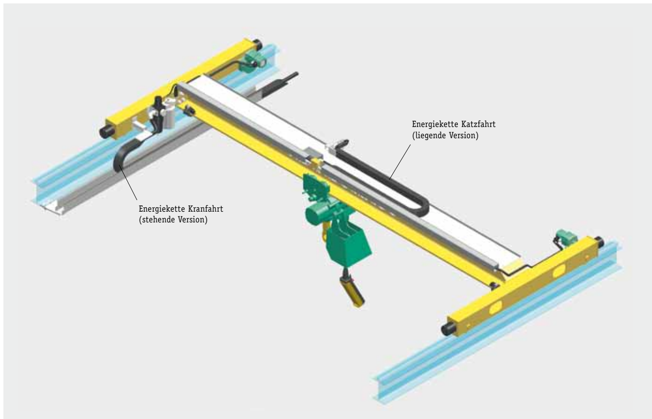
Energiezuführung an einem Laufkran
