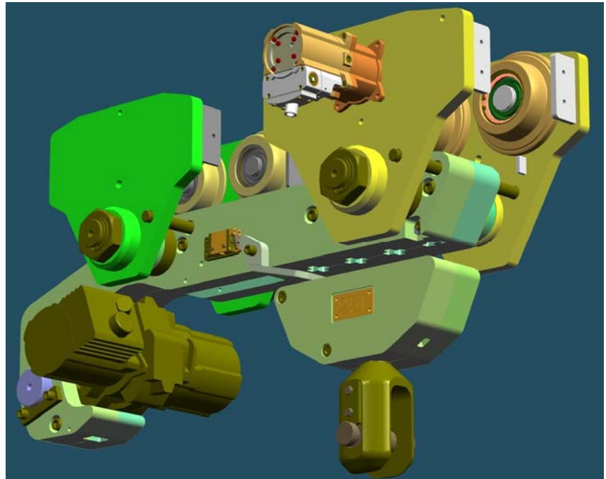
CAD-Modell der neuen JDN-Flachlaufkatze LMF 25 t
